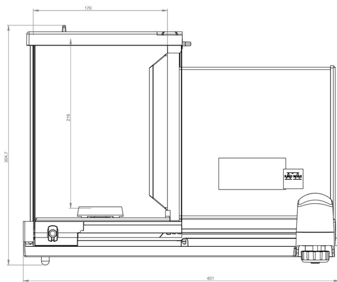
XA 6/21.5Y.M.A Microbalance
