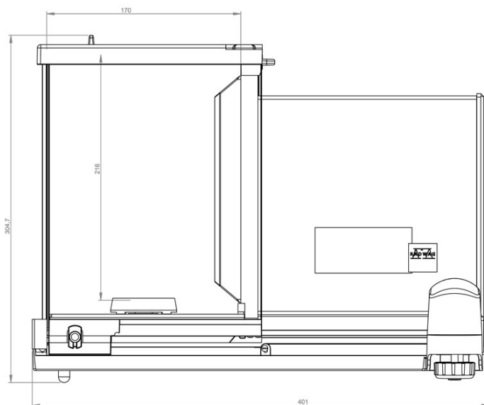
XA 6.5Y.M.A Microbalance
